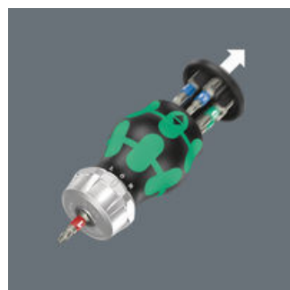
Grebet kan åbnes og giver således adgang til de seks bits inde i magasinet.
